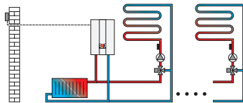
Módulo de ampliación KM-2
